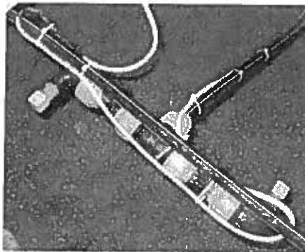
Varmekabel i biofilteret
