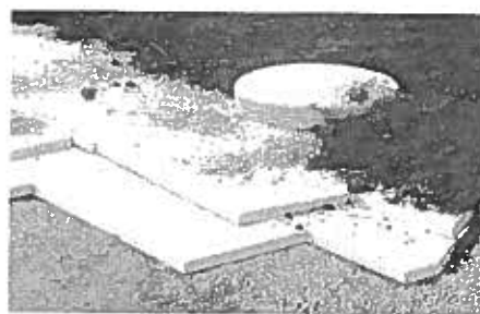
Frostsikring av tanker
